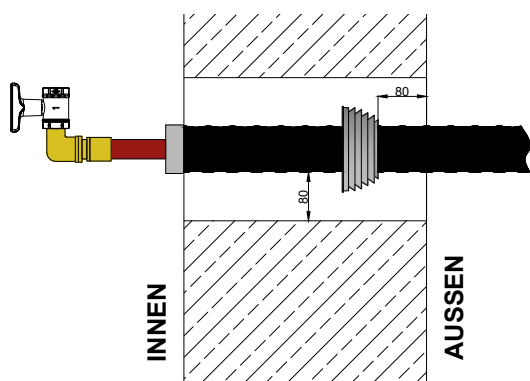
Abb. 41: Montageempfehlung Labyrinthdichtung
