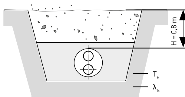
Abb. 23: Rohrgraben double-Rohr
