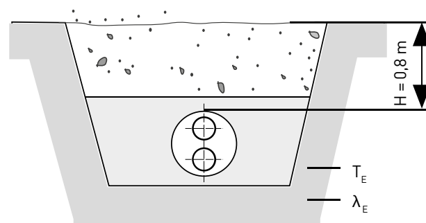
Abb. 25: Rohrgraben double-Rohr
