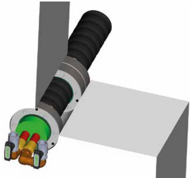
Abb. 48: Dichtflansche CaldoSEAL DW60 und NDW30 eingesetzt
