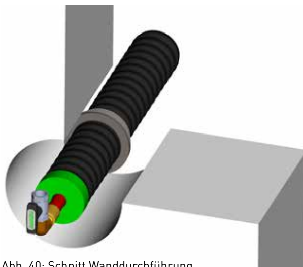
Abb. 40: Schnitt Wanddurchführung
