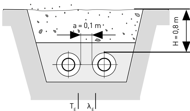
Abb. 20: Rohrgraben single-Rohr
