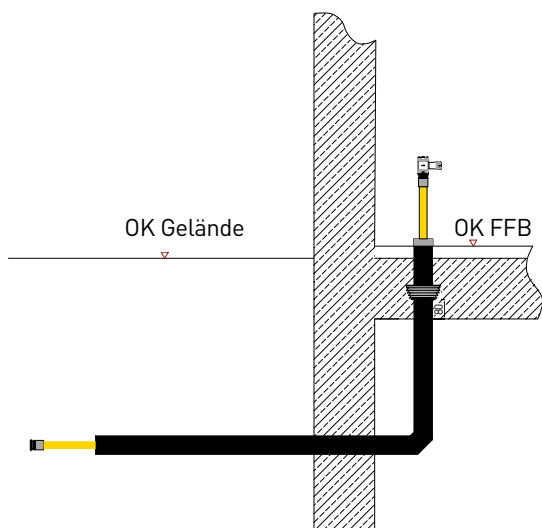
Abb. 52: Einbaubeispiel Hauseinführungsbogen
