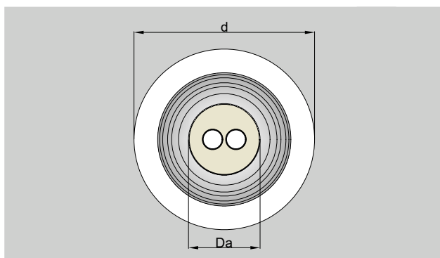
Abb. 39: Kernlochbohrung FibreFLEX/CaldoPEX double
