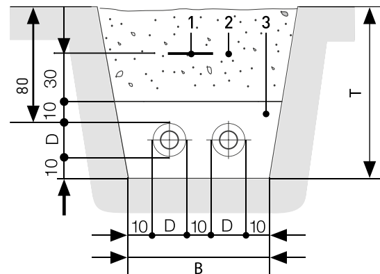
Abb. 32: Grabenquerschnitt 2 Rohre
