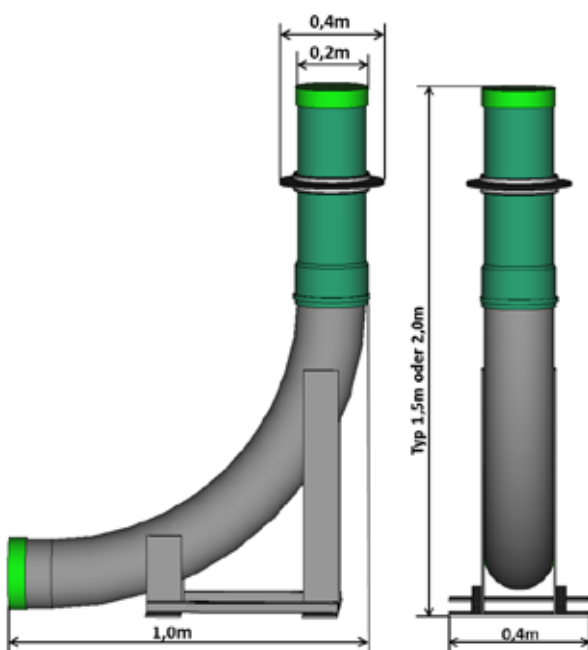
Abb. 55 ENERPIPE Leerrohrbogen Maße
