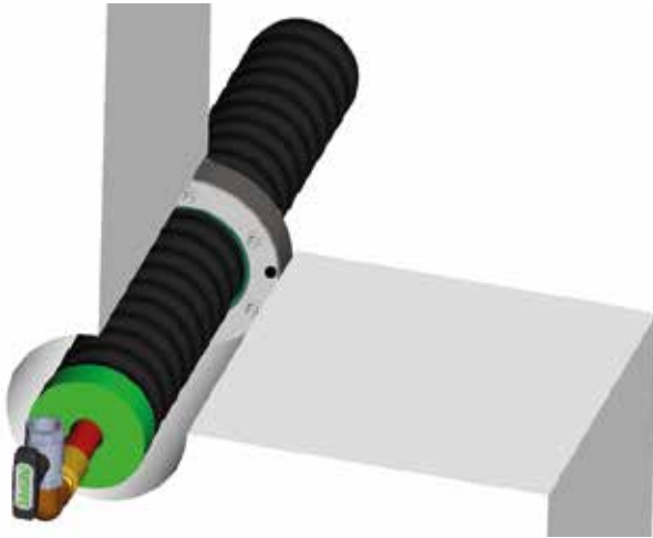
Abb. 46: Dichtflansch CaldoSEAL NDW30
