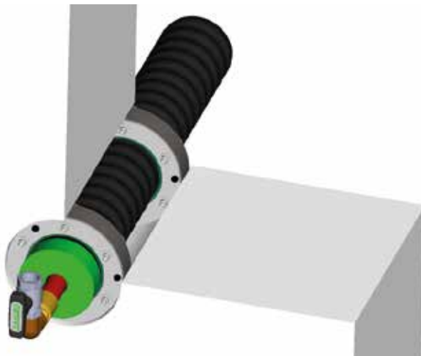
Abb. 47: Dichtflansch CaldoSEAL NDW30, zwei Mal eingesetzt bei Wandstärke \geq 25 cm
