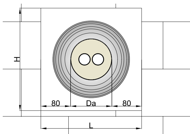
Abb. 37: Mauerdurchbruch FibreFLEX/CaldoPEX double
