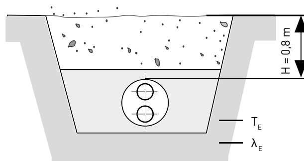
Abb. 21: Rohrgraben double-Rohr
