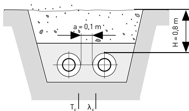
Abb. 24: Rohrgraben single-Rohr
