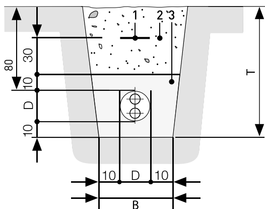
Abb. 31: Grabenquerschnitt 1 Rohr
