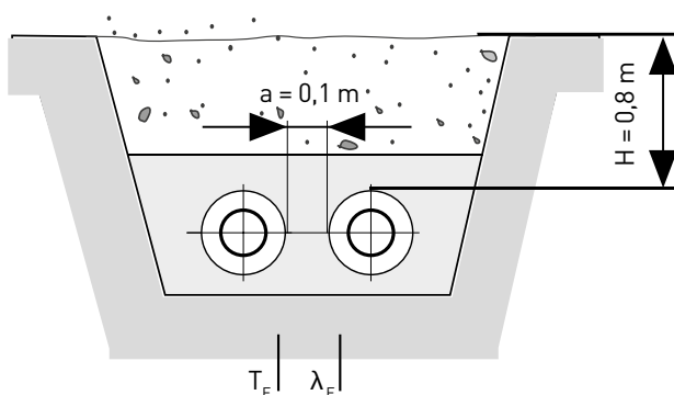
Abb. 22: Rohrgraben single-Rohr
