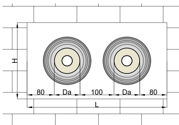
Abb. 36: Mauerdurchbruch FibreFLEX/CaldoPEX-Rohr single
