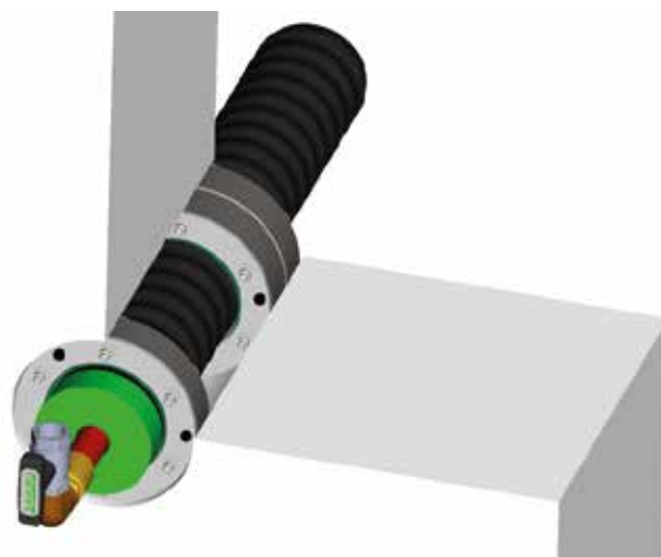
Abb. 45: Dichtflansch CaldoSEAL DW60 und NDW30 bei Wandstärke \geq 25 cm
